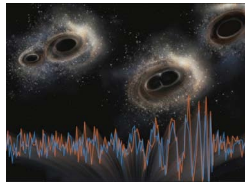
Rappresentazione della sequenza della fusione dei due buchi neri e il segnale rilevato.
